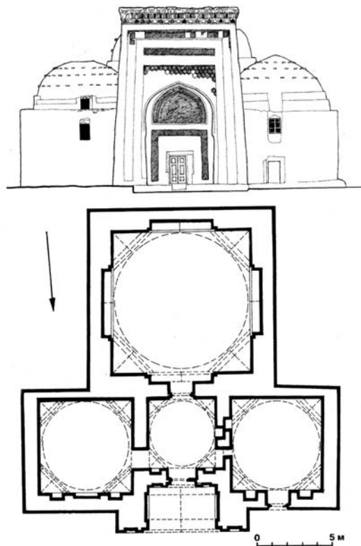
Куня-Ургенч. Мавзолей Наджм ад-Дина Кубра. Северный фасад и план (по И.И.Ноткину)
