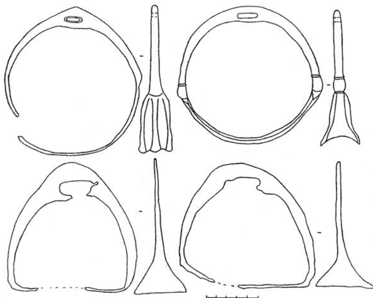
Стремена. Железо. Укек. XIII–XIV вв. НМ РТ (по И.Л.Измайлову, Л.Ф.Недашковскому)
