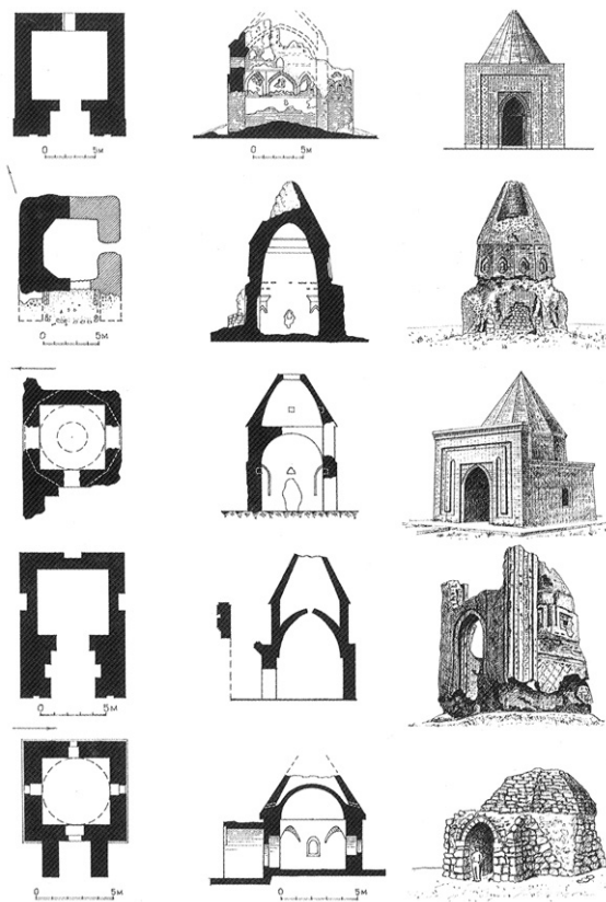
Типы мавзолеев – кешене. Приаралье. XIII–XIV вв.
