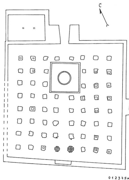
План мечети. Большие Кучугуры (по Е.А.Армарчук)
