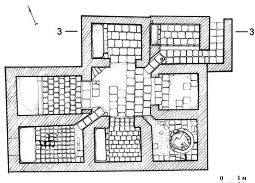
Городище Антоновка. План усадьбы богатого человека
