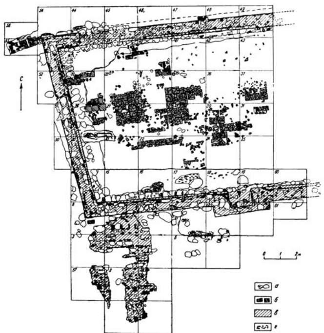
План Большой мечети Верхнего Джулата (по О.В.Милорадович) а – камни, б – кирпичи, в – цементирующий раствор, г – уголь
