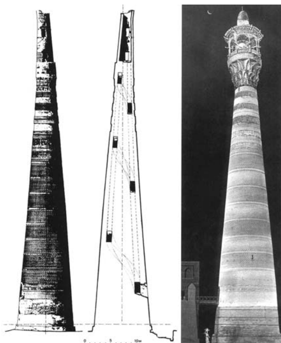
Куны-Ургенч. Минарет Кутлуг-Тимура. Южный фасад и разрез по обмерам А.Н.Виноградова. Справа – реконструкция В.Н.Артемьева
