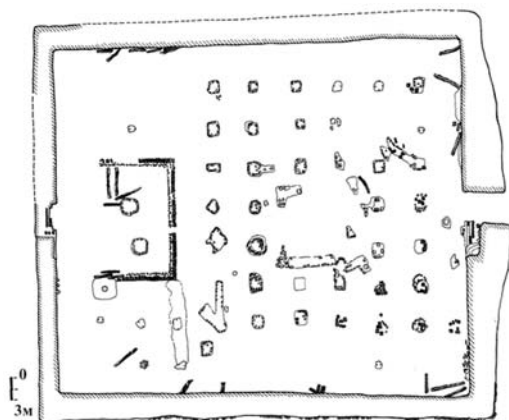
Городище Антоновка. План мечети
