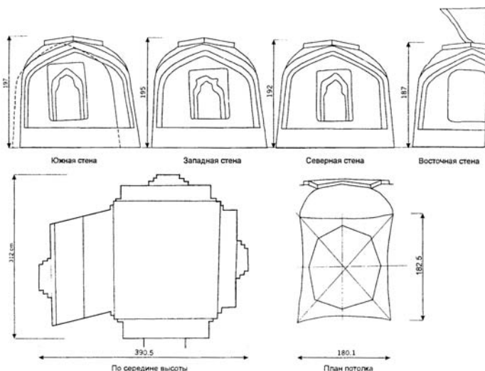
Подземный склеп-мавзолей Нижнего Джулата. План
