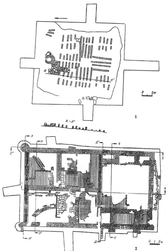
Планы бани и медресе. Большие Кучугуры (по Е.А.Армарчук)
