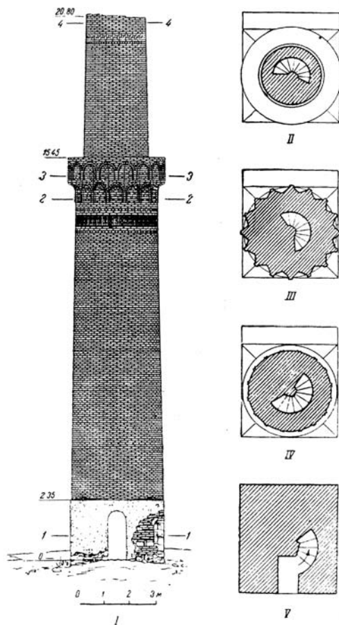
Татартупский минарет (по О.В.Милорадович)
