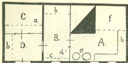
Рис. 43. План бани кулака: А—баня; В—чистый передбанник; С—помещение с постелью; Д—передбанник; а—нары; b—лавка; с—шест; d—угольник для комода; e—кадки с водой; f—полк для парня
