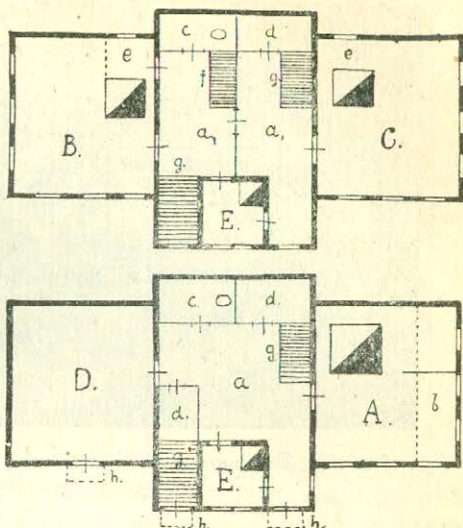
Рис. 27. План двухэтажного дома с крестообразным планом. А—черная изба; В—чистая изба; С—жилая чистая половина; Д—кладовая; Е—комната для старух; а—хозяйств. сени; а 1 —чистые сени; в.—нары; с—уборная; d—чулан; е—комната для омовений; f—лестница на чердак; g—лестница наверх; h—навес над входом.
