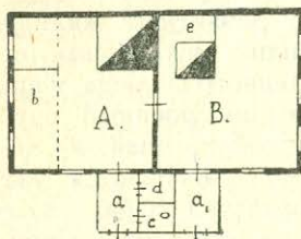
Рис. 26. План пятистенника, (анотац. см. 27).
