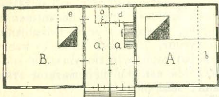
Рис. 25. План „шестистенника“ (анотац. см. 27).
